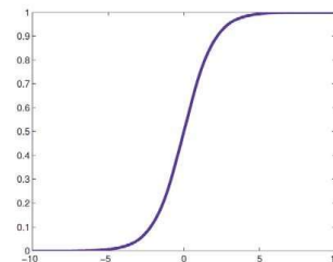
SIGMOID FUNCTION
